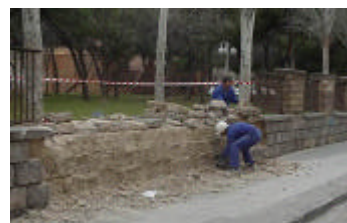
Demolición muro
